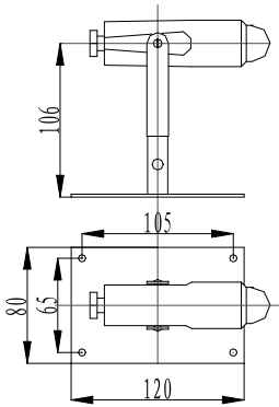
光控探头结构示意图
